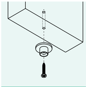
Pivot inferior Fixação ao ripado
